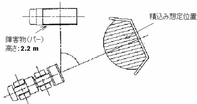
図4 掘削位置と積み込み位置の関係
