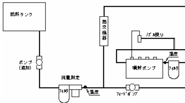
図 1 直接消費流量測定方法
