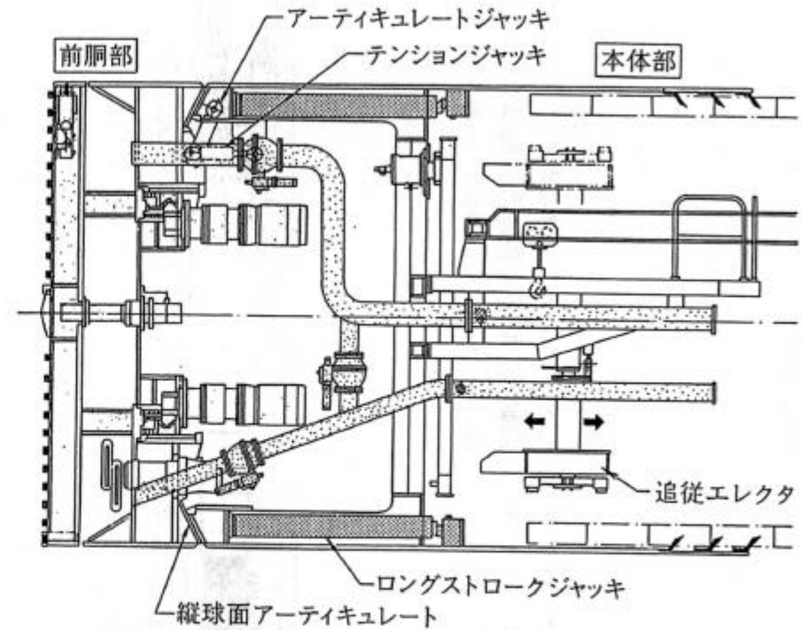
F-NAVI シールド機の構造
