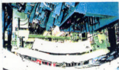
③正確な位置決め機能を持つ セグメント供給装置
