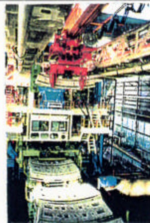
④1リング分110個のナット ストックと正確な供給を可能 とするナット供給装置
