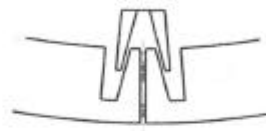
① コッタ継手セグメントの自動組立試験
