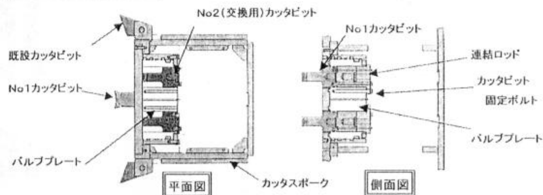
交換ビット取付構造
