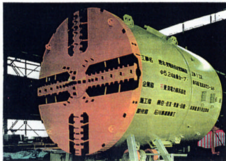
港北変電所新設工事
