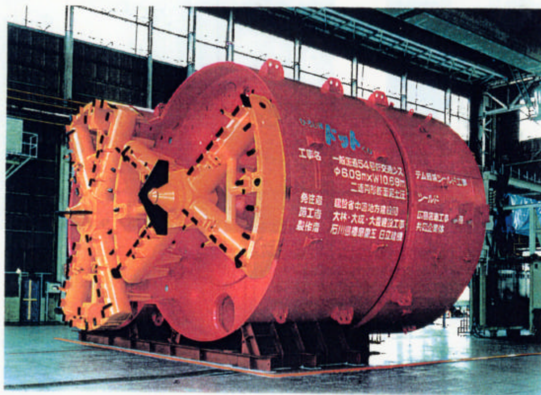
広島新交通システム 外径φ6.09×巾10.69m
