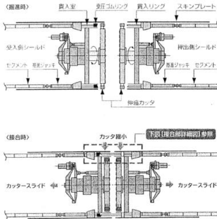
地中接合機構図
