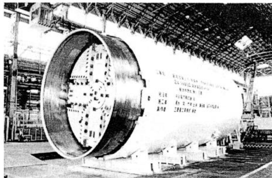
貫入リング側シールド
