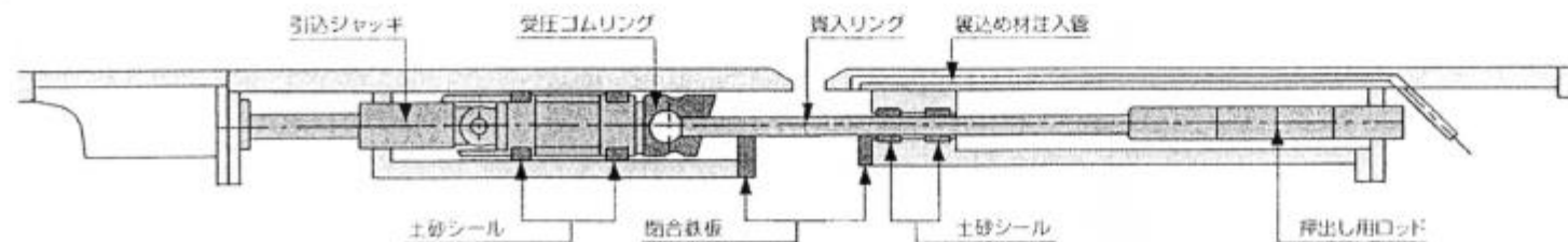
接合部詳細図
