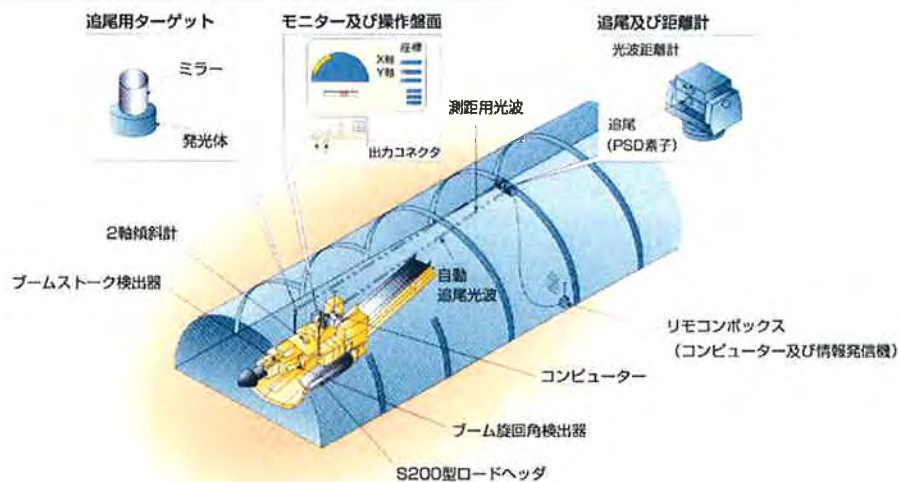
施工例
